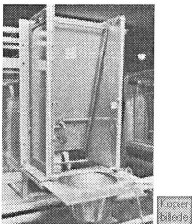
Figur 1. Opsamlingsbur til fordøjeligheds- og balanceforsøg med svin. Grisens adgang til fodertruget reguleres med den lodrette plade. Fodertruget er aftageligt.
