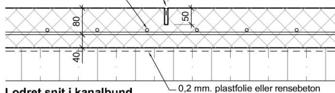
Lodret snit i kanalbund
