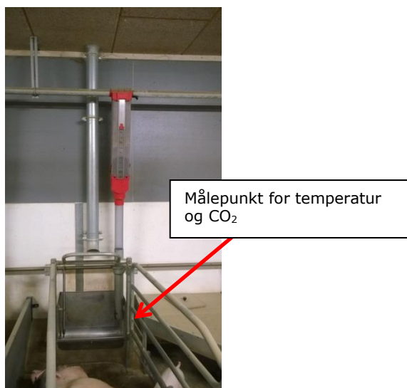
Figur 2. Placeringen af temperatur- og CO 2 -sensorer. Placering af målepunkt for logning af temperatur og CO 2 . Følerne blev placeret for enden af et jernrør for at beskytte følere og ledninger.
